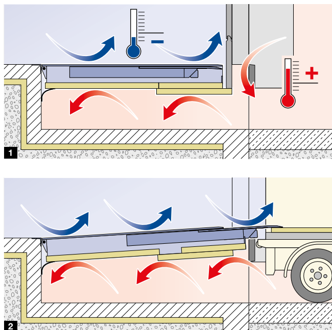
Déperditions thermiques* par an au niveau de la plateforme et de la lèvre A une différence de température de 20 °C
