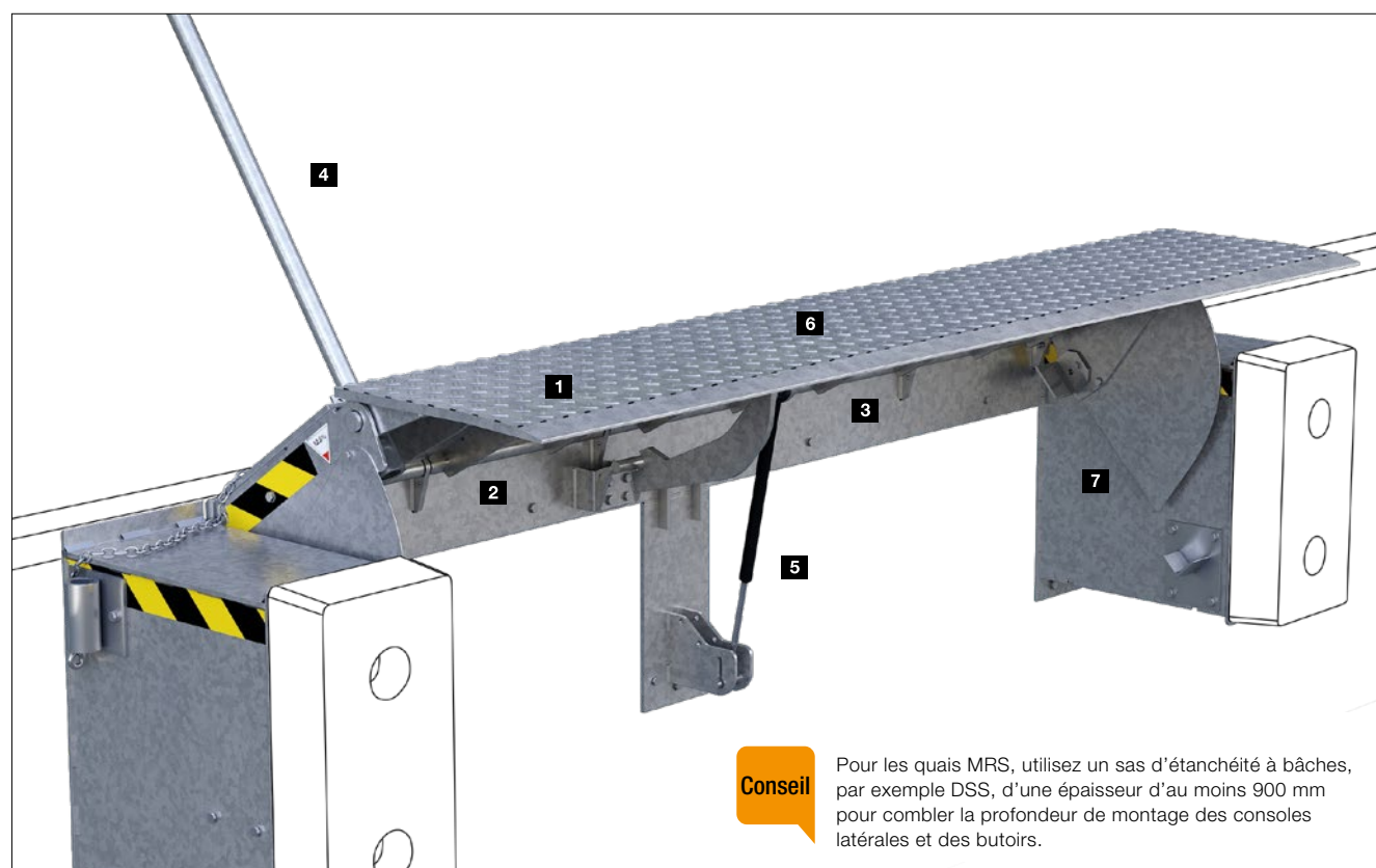
Niveleur de quai mécanique MRS-V en exécution galvanisée
