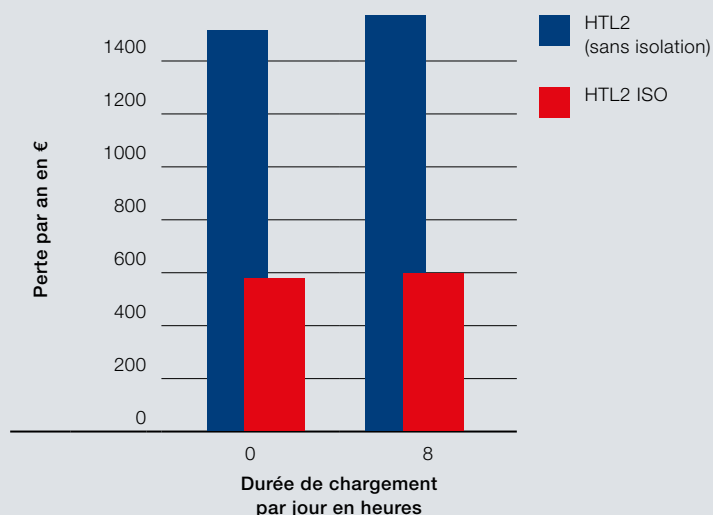
Déperditions thermiques* par an au niveau de la plateforme et de la lèvre A une différence de température de 20 °C
