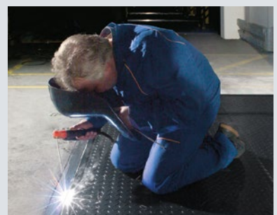
Soudage au niveau des cornières périphériques – Terminé.
