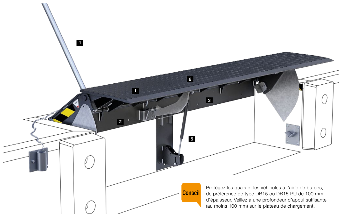
Niveleur de quai mécanique MLS en noir trafic RAL 9017
