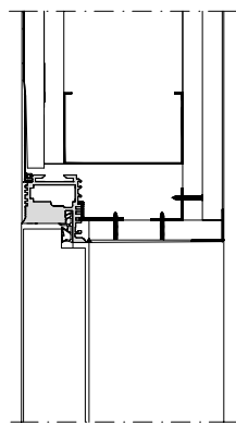
Coupe verticale ouverture normale vers l'extérieur (type NA)
