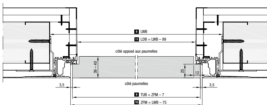
Coupe horizontale type NA avec vantail de porte à ouverture classique
