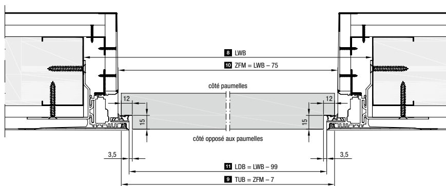
Coupe horizontale type RI avec vantail de porte à ouverture inversée
