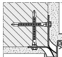
Pose avec pattes d'ancrage à cheville
