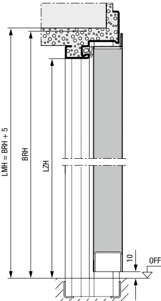
Coupe verticale
