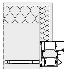
Huisserie à rupture de pont thermique Montage rapide
