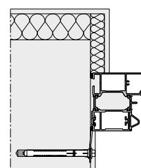
Huisserie tubulaire pour pose dans la baie (profilé 21101)
