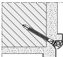
Huisserie d'angle spéciale Montage par vis traversantes au travers de la rainure
