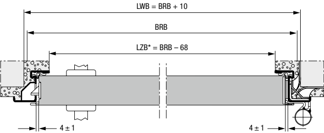
Coupe horizontale
