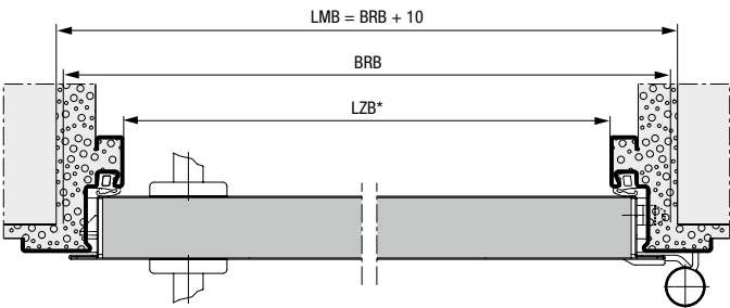
Coupe horizontale
