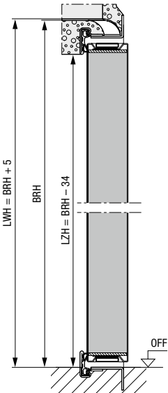
Coupe verticale
