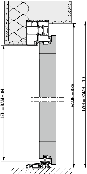
Coupe verticale
