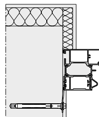
Huisserie à rupture de pont thermique Montage par pattes d'ancrage
