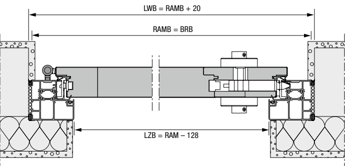
Coupe horizontale
