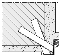
Pose avec patte d'ancrage
