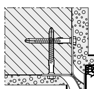
Pose avec pattes d'ancrage à cheviller
